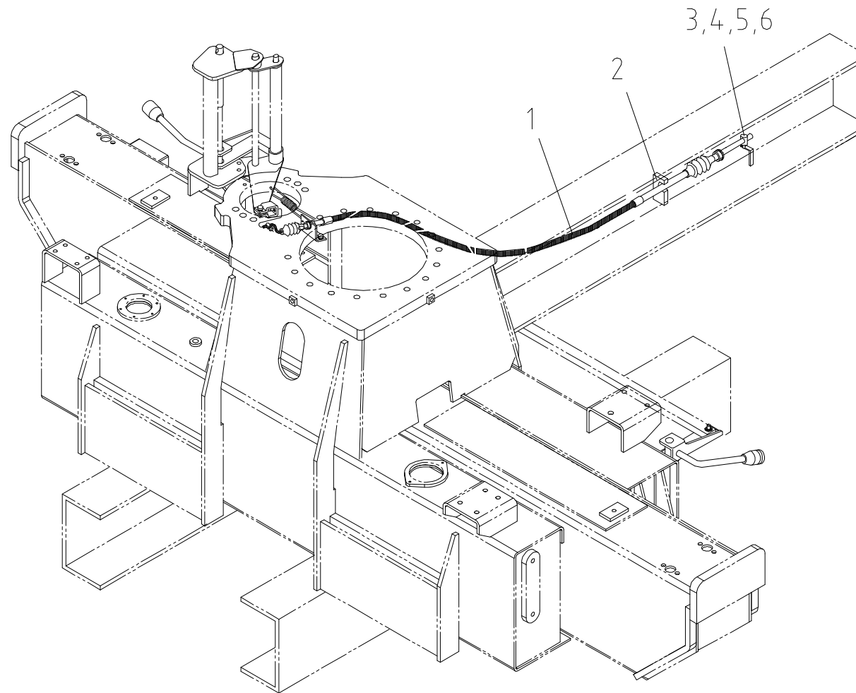
악셀 시스템 파트 Fig. 8-3 SCS513 ACC' SYSTEM PART
