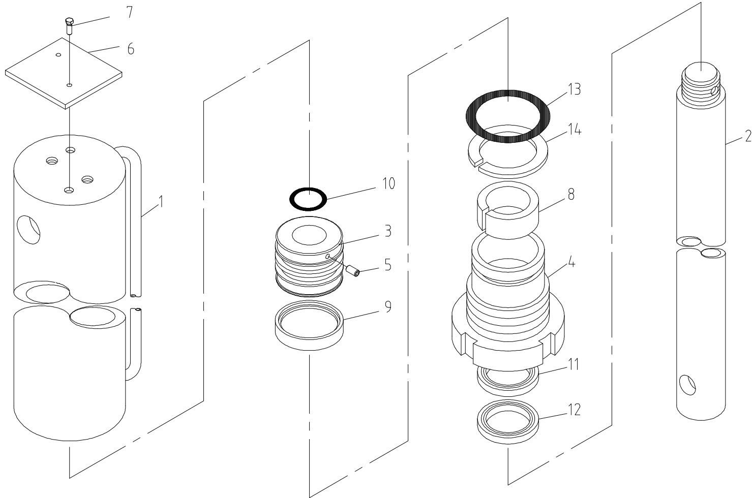
잭 실린더 조립체 Fig. 4-1 SCS513 JACK CYL' ASS'Y
