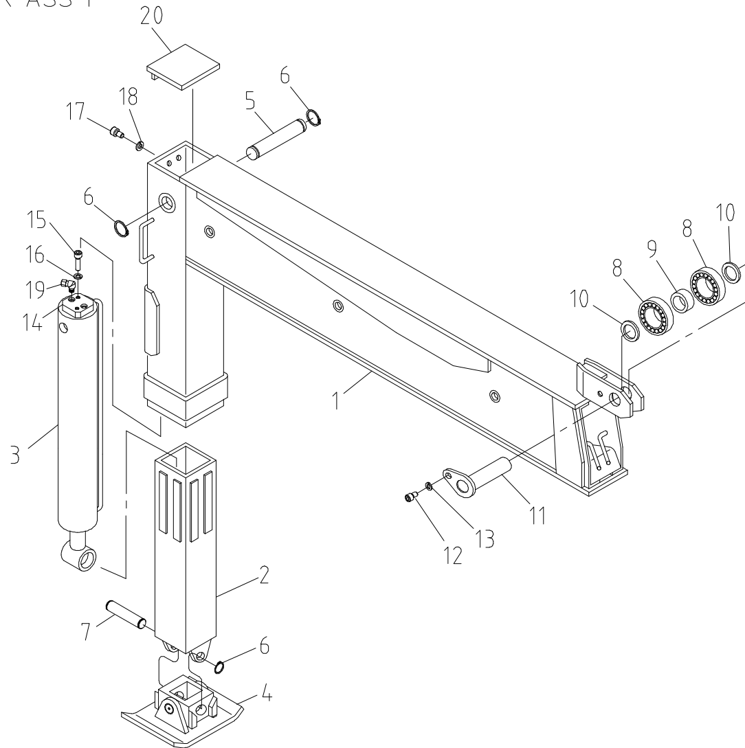
아우트리거 조립체 (대우 16톤용) Fig. 4 SCS513 OUTRIGGER ASS'Y
