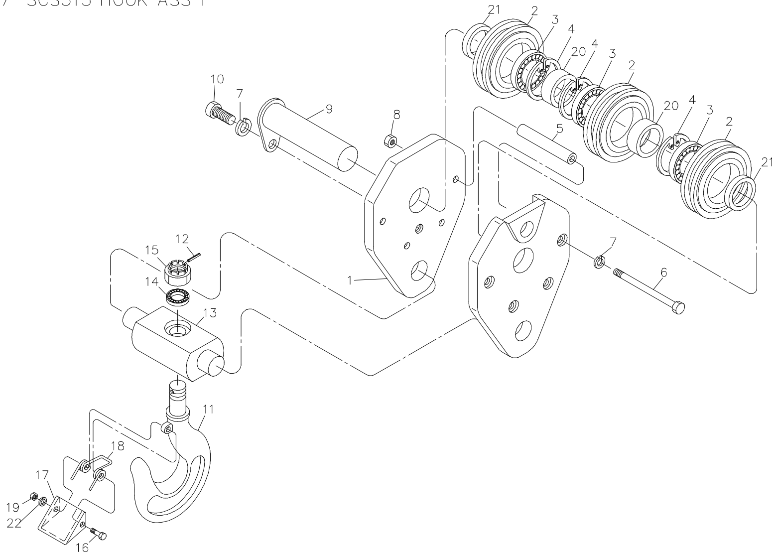
후크 조립체 Fig. 7 SCS513 HOOK ASS'Y
