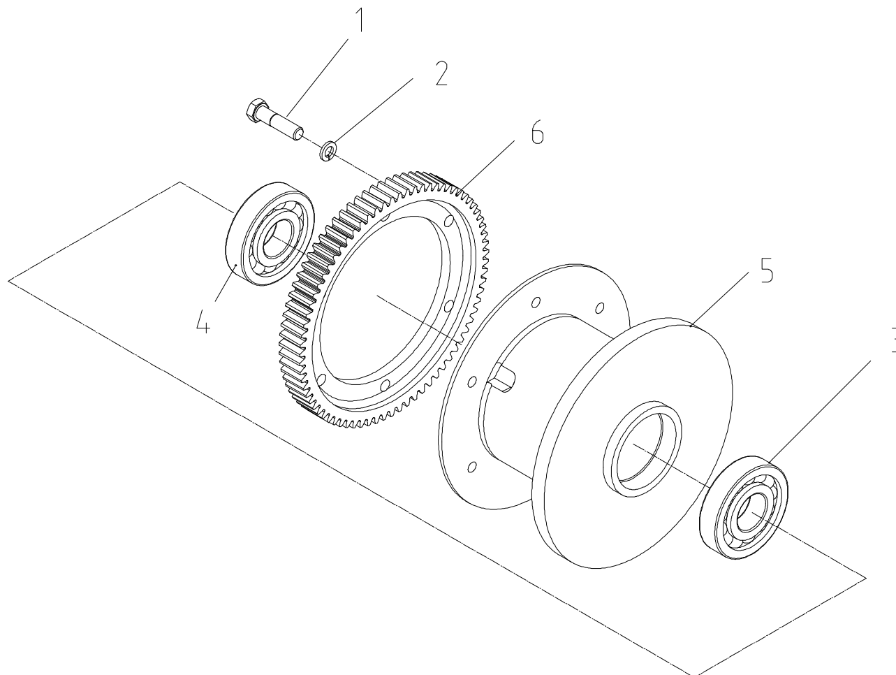
드럼 조립체 Fig. 2-1 SCS513 DRUM ASS'Y
