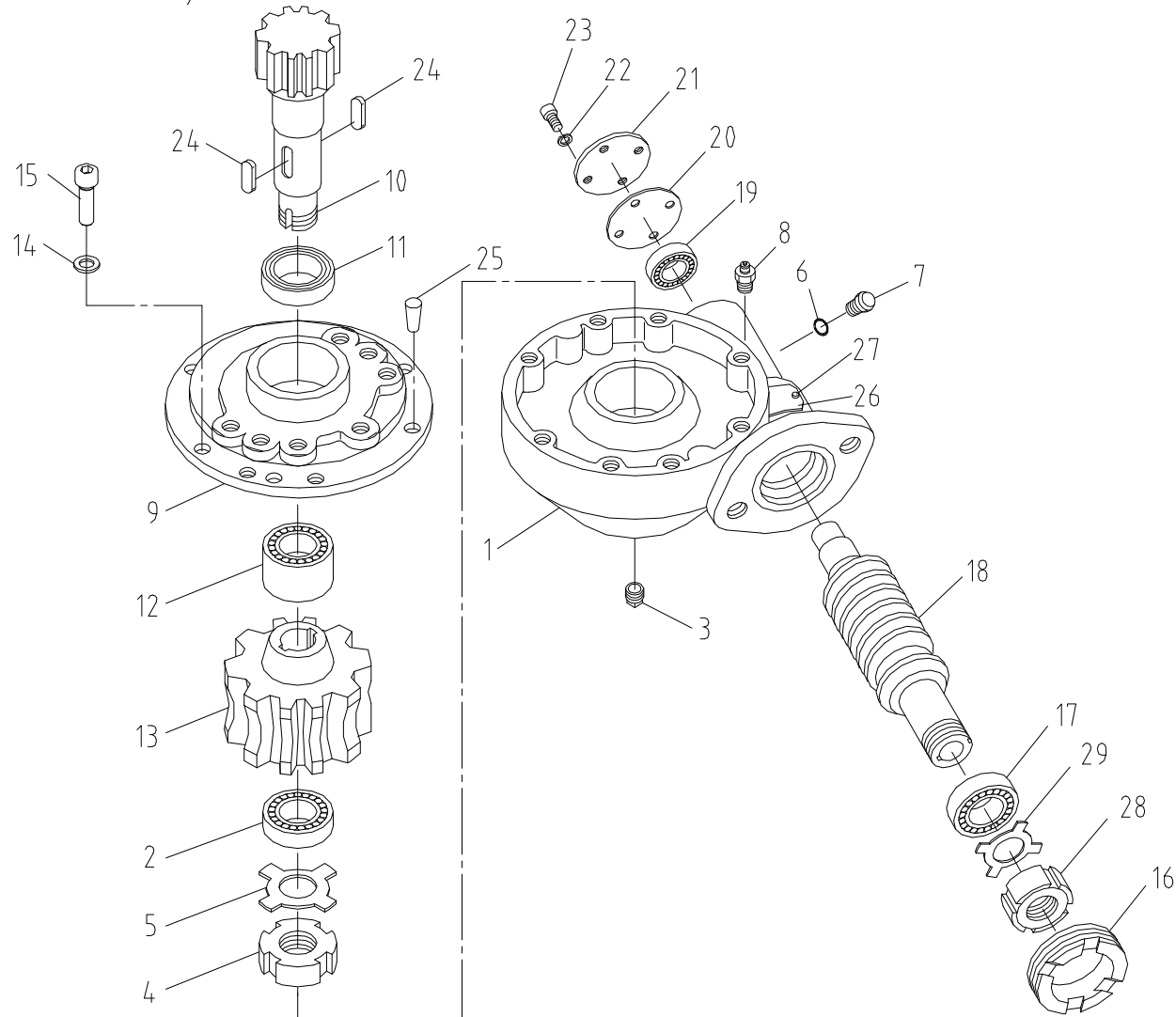
스윙 감속기 셋트 Fig. 3-1 SCS513 SWING R/G SET
