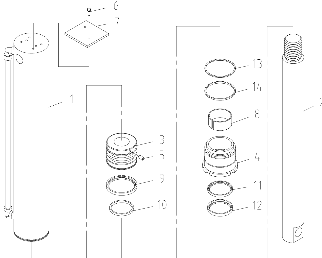
잭 실린더 조립체 (대우 16톤용) Fig. 4-1 SCS513 JACK CYL' ASS'Y
