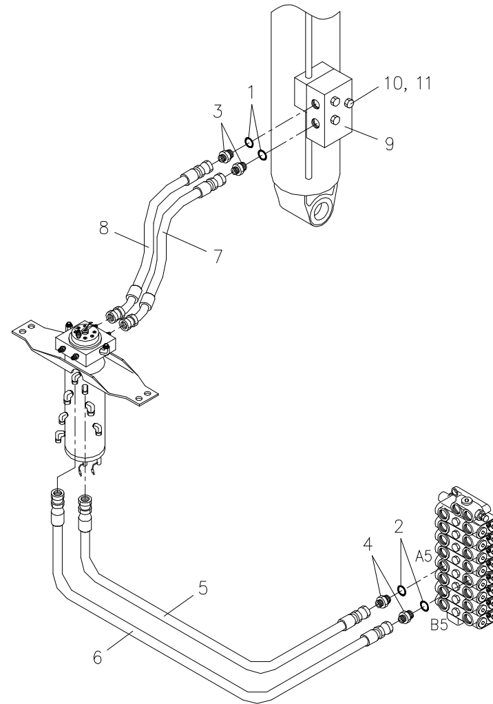
데릭 배관 Fig. 5-2 SCS513 DERRICK PIPING
