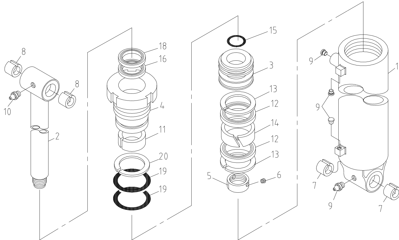
데릭 실린더 조립체 Fig. 2-3 SCS513 DERRICK CYLINDER ASS'Y
