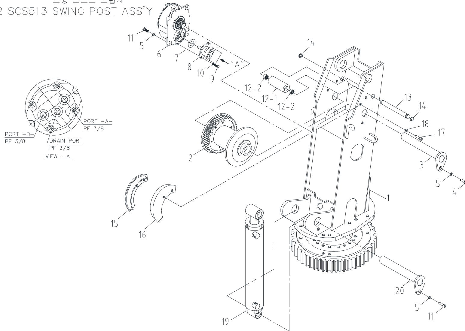
스윙 포스트 조립체
