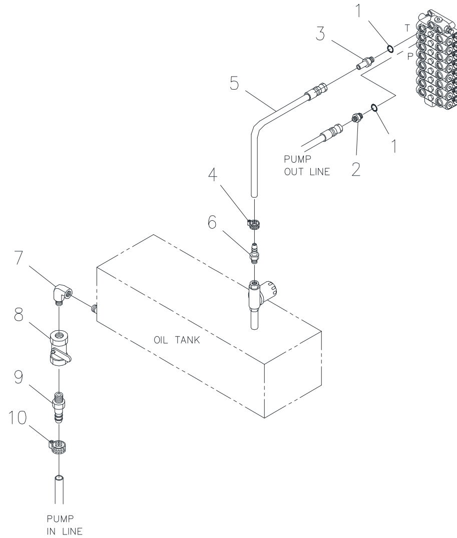
디스트리뷰터 배관 Fig. 5-1 SCS513 DISTRIBUTOR PIPING
