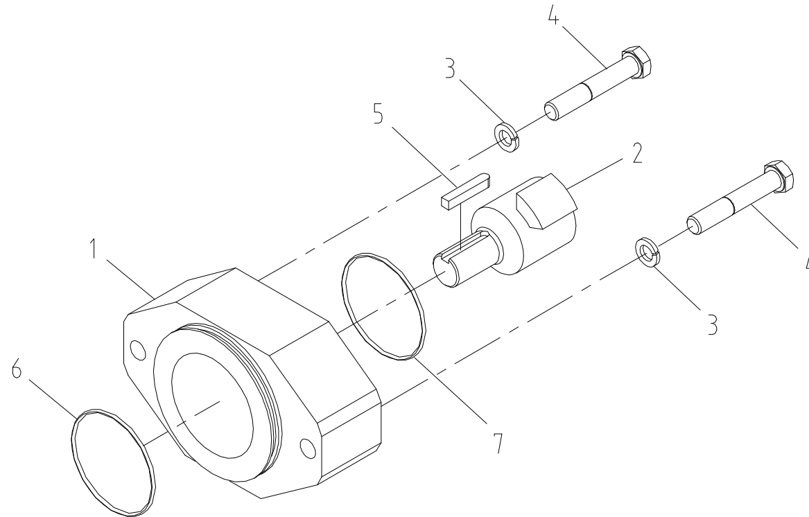
스윙 감속기 아답터 조립체 Fig. 3-2 SCS513 SWING R/G ADAPTER ASS'Y
