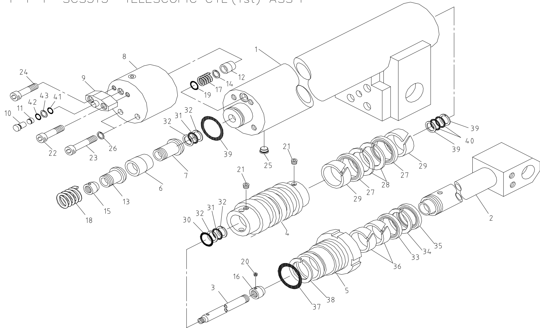
텔레스코픽 실린더(1단) 조립체 Fig. 1-1-1 SCS513 TELESCOPIC CYL'(1st) ASS'Y
