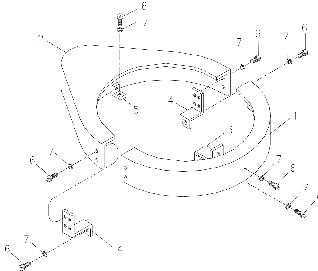
스윙 커버 조립체 Fig. 3-5 SCS513 SWING COVER ASS'Y
