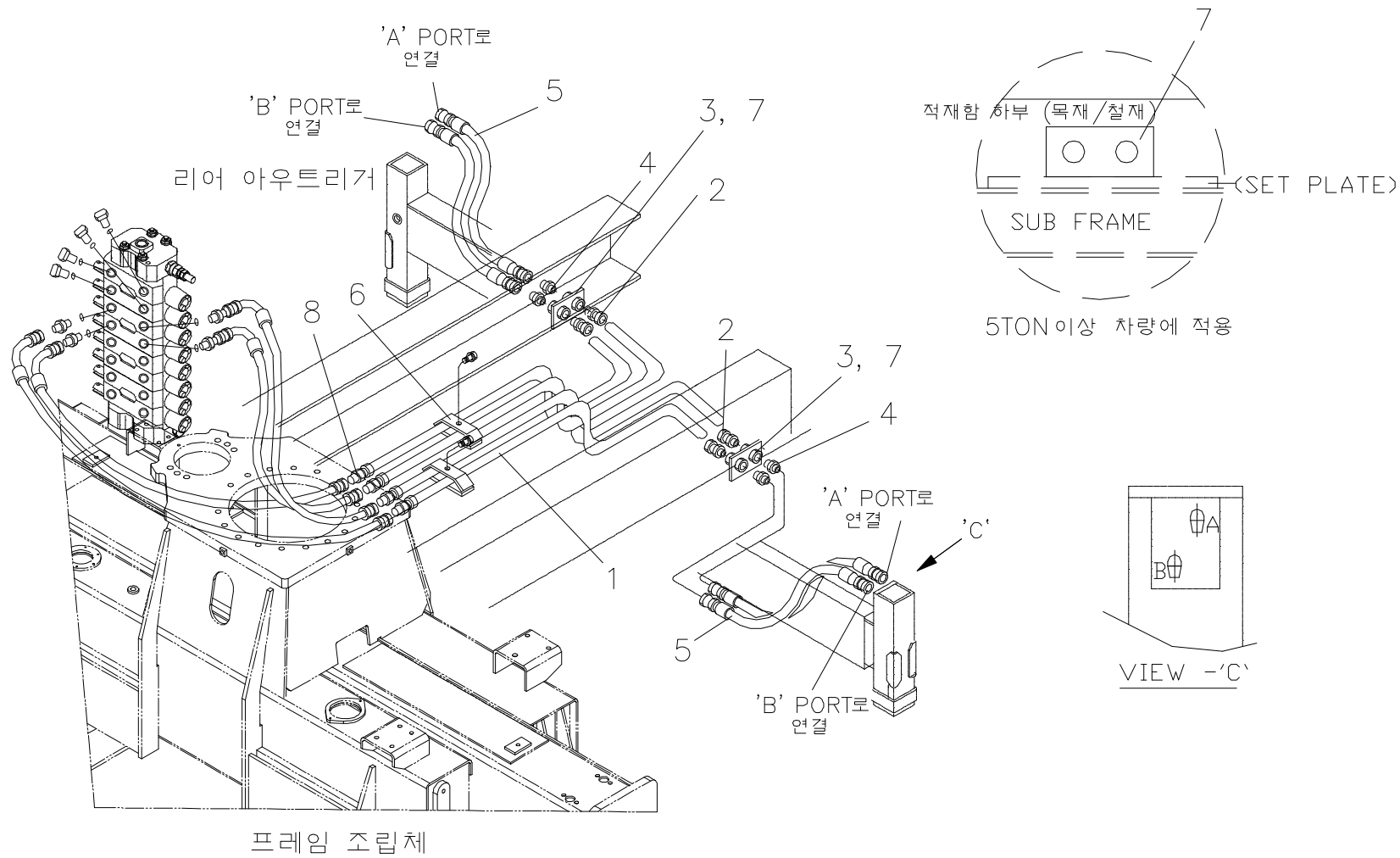
후방 장착 배관 파트 Fig. 8-4 SCS513 R/O M/T PIPING PART
